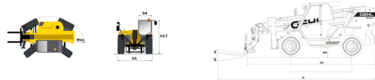
TX 4017 - Diagrama dimensional
